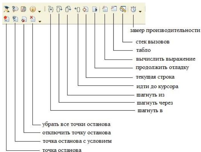
Рис. 24. Панель отладки
