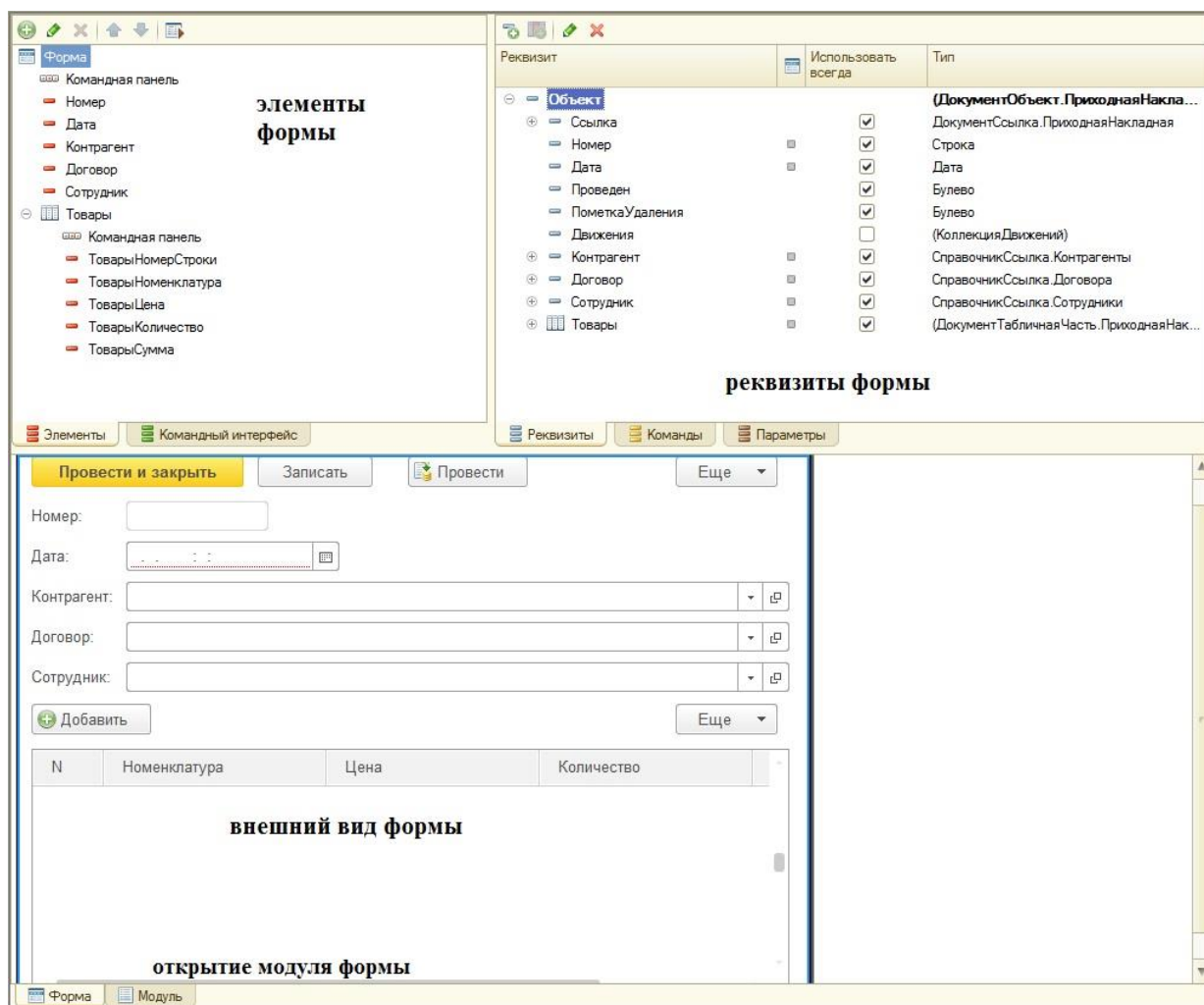
Рис. 30. Конструктор формы
