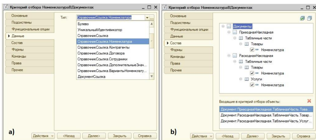
Рис. 60. Критерий отбора
